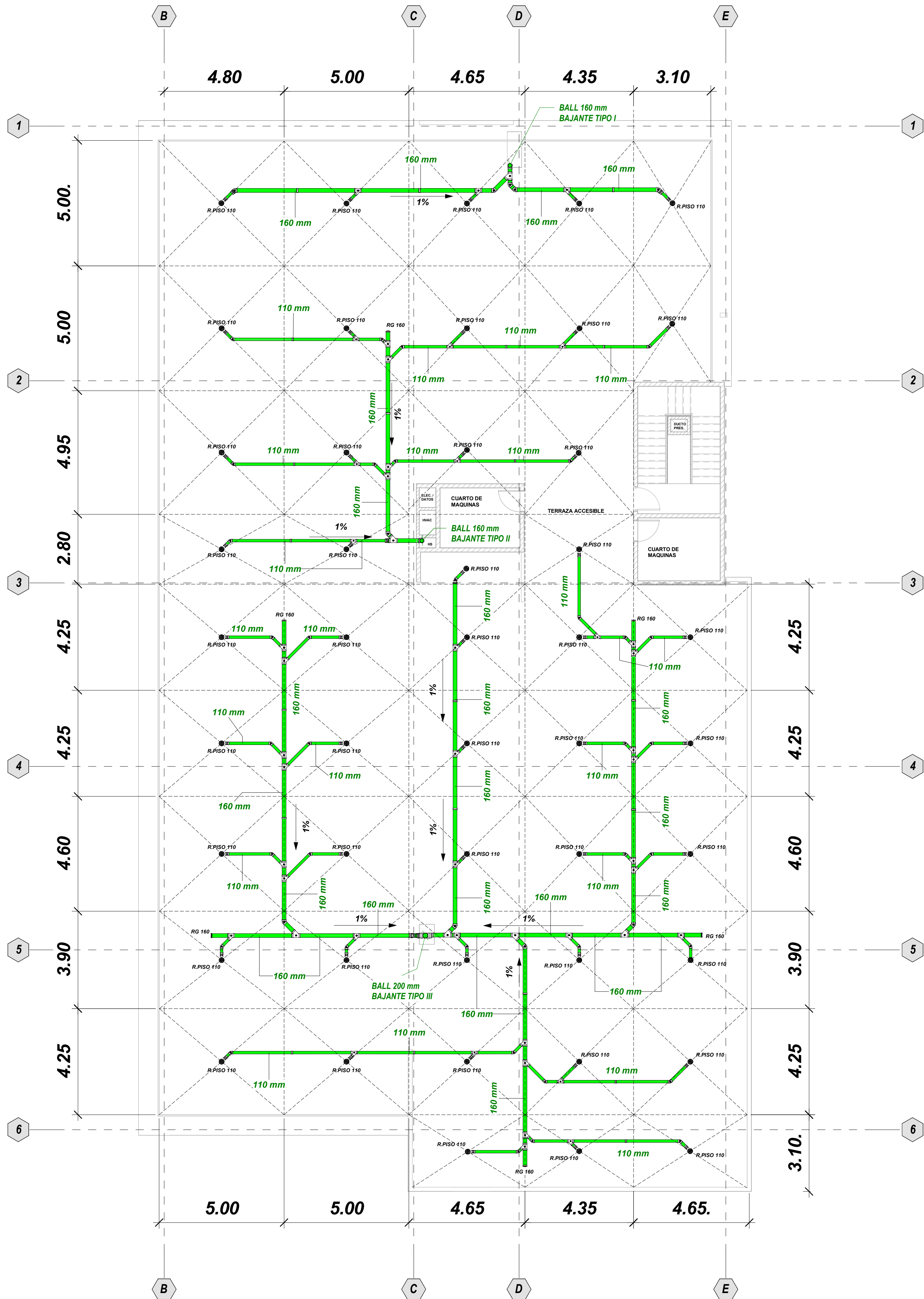
1 2 - PISO 8 - ALL / N+32.64 1 : 100
