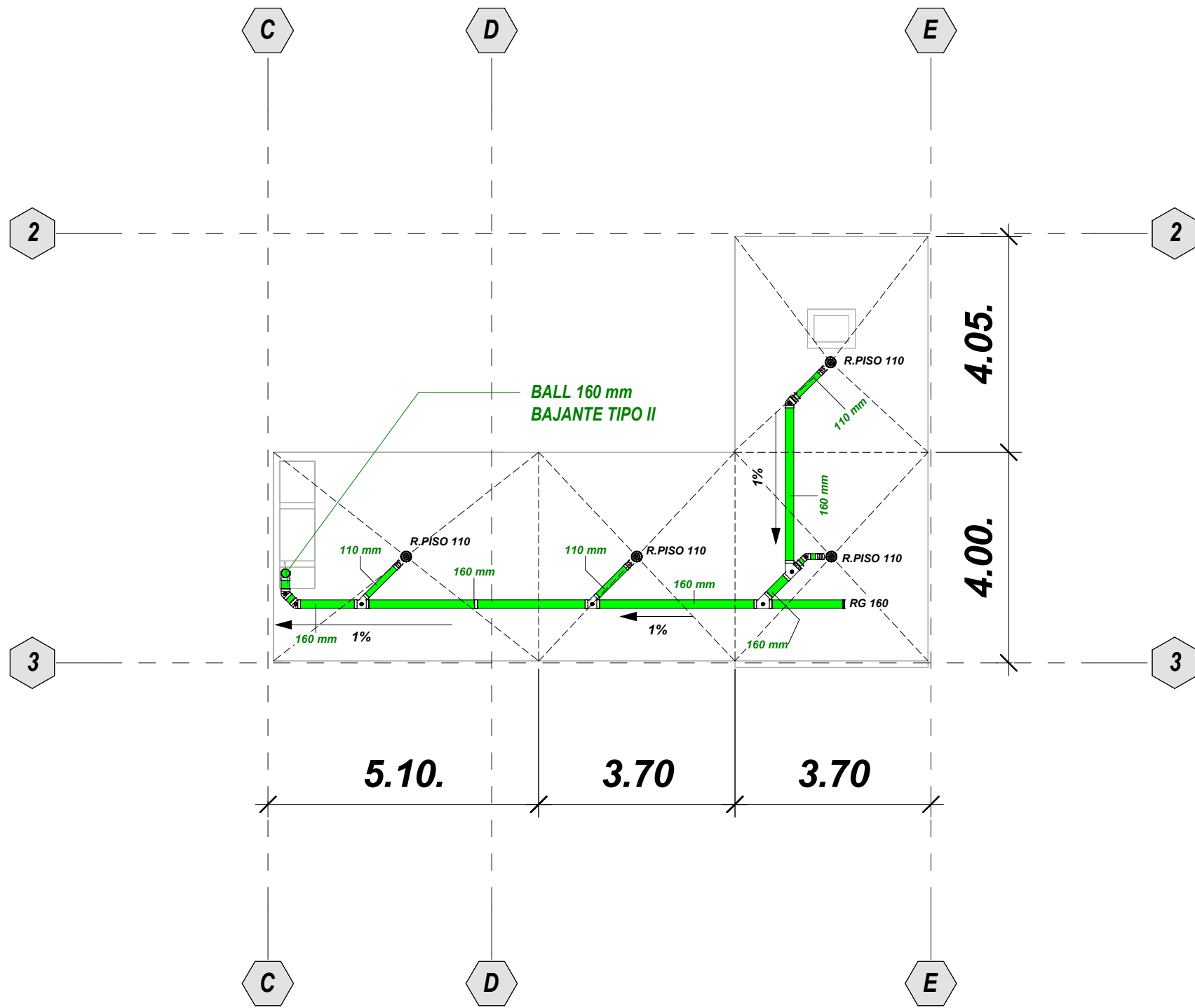
2 1 - PISO 9 - ALL / N+36.72 1 : 100
