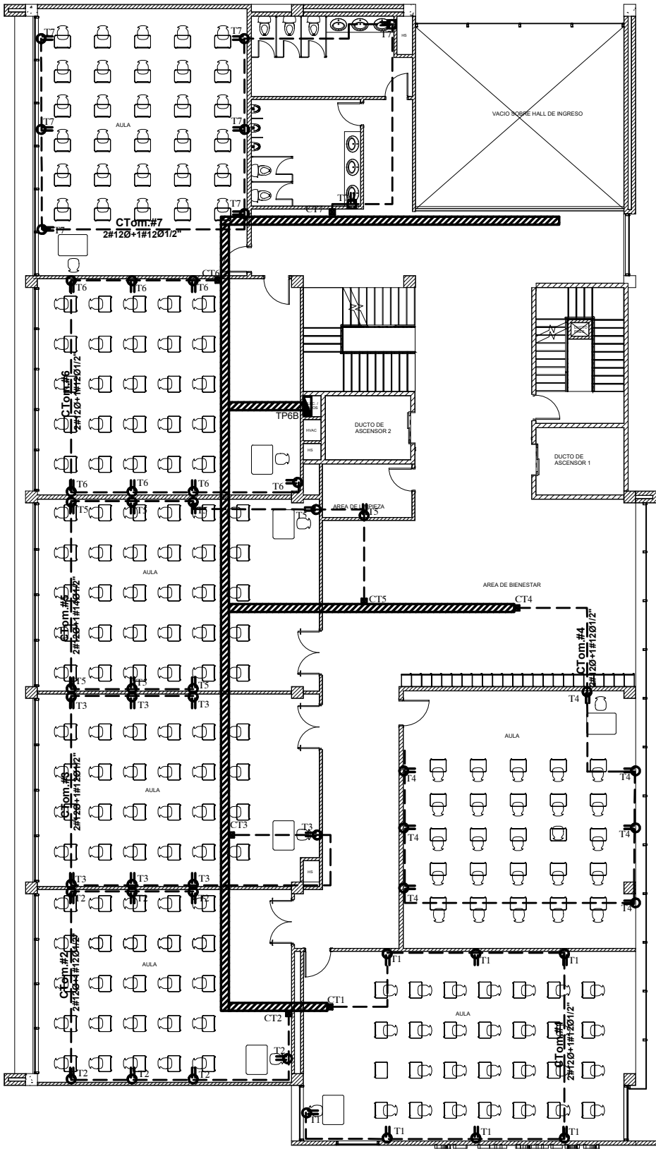
SEPTIMA PLANTA ALTA NV.+28.56
