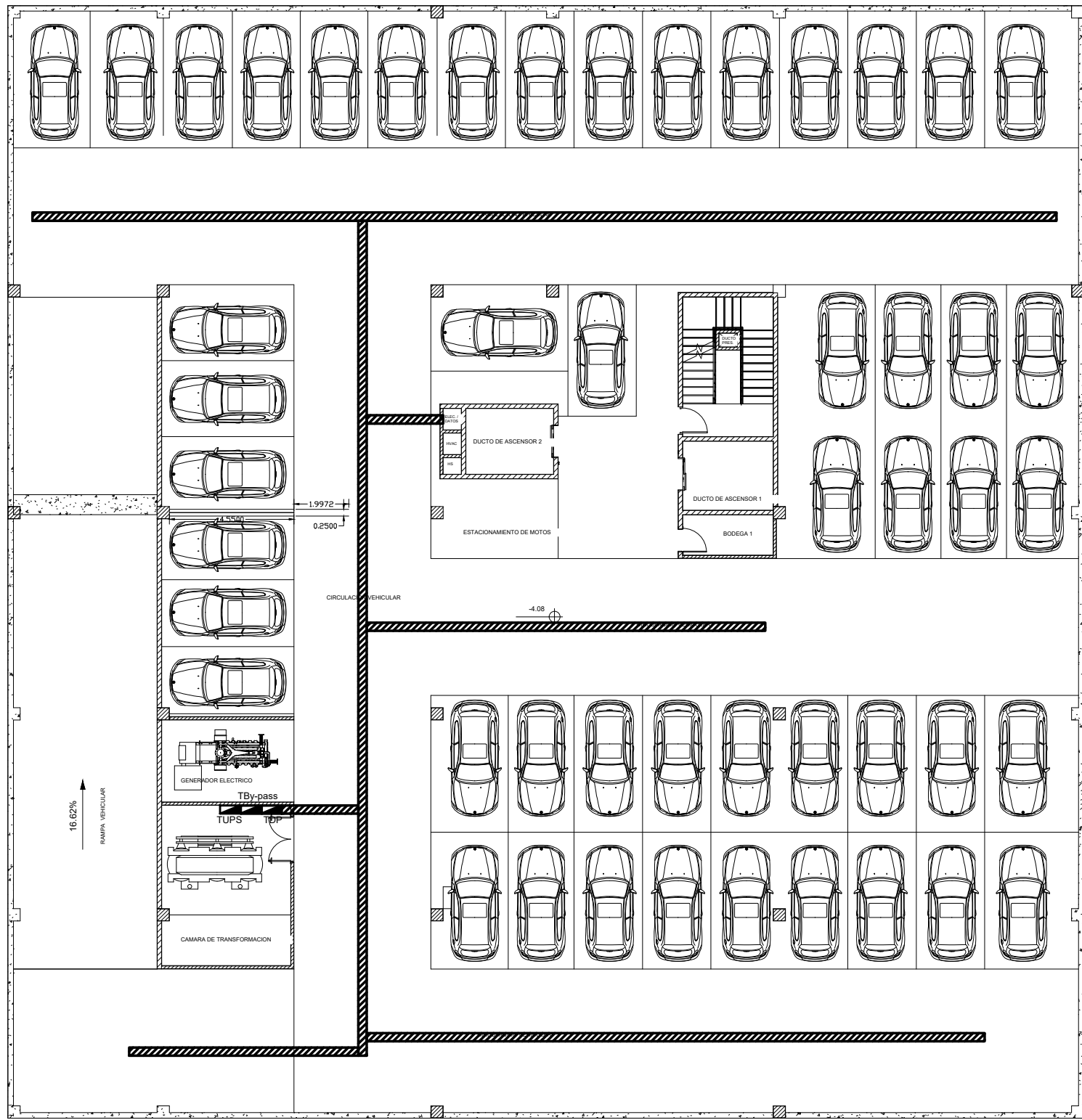
SUBSUELO 1 NV.-4.08
