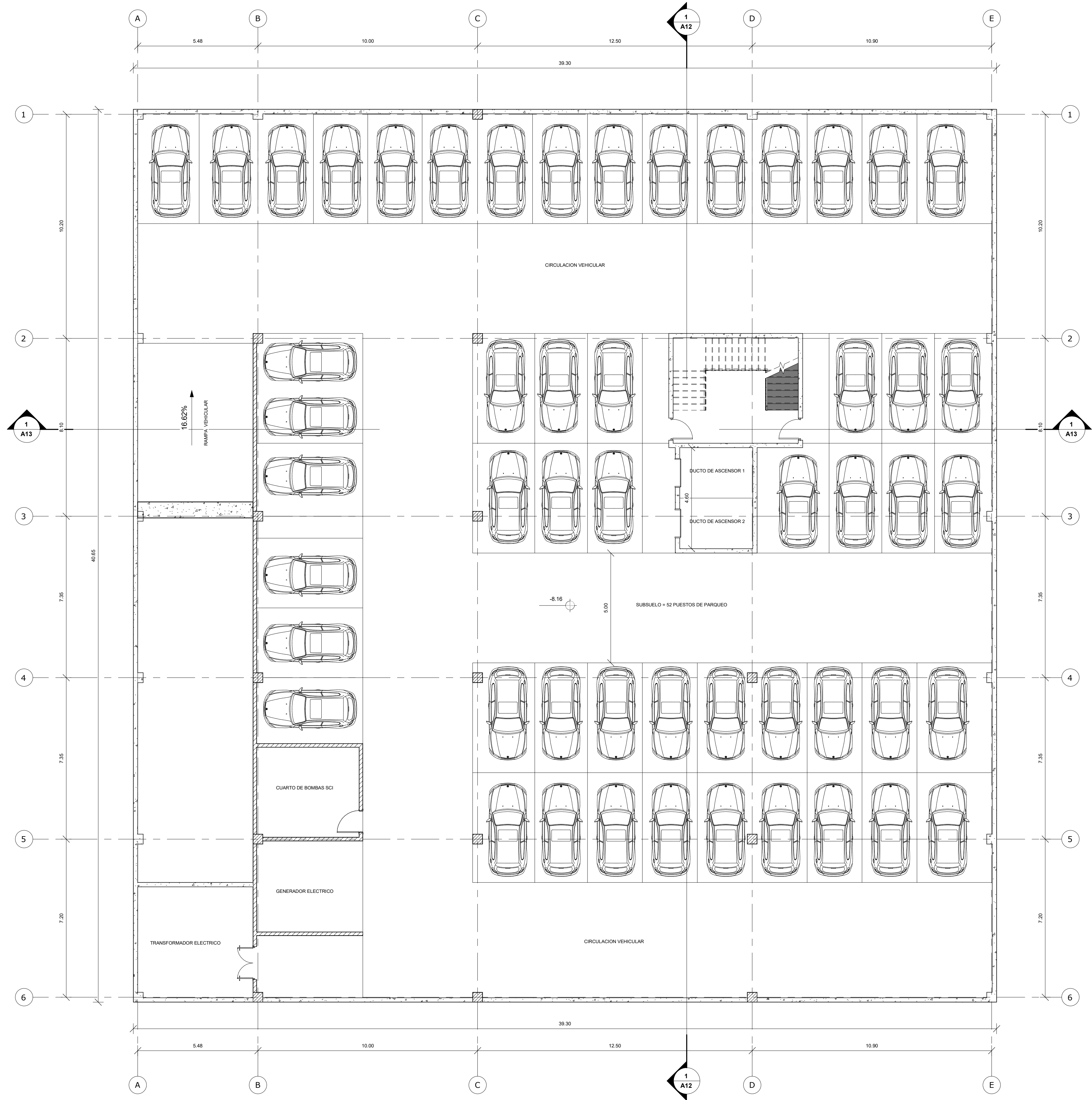
1 SUBSUELO NIVEL -8.16
