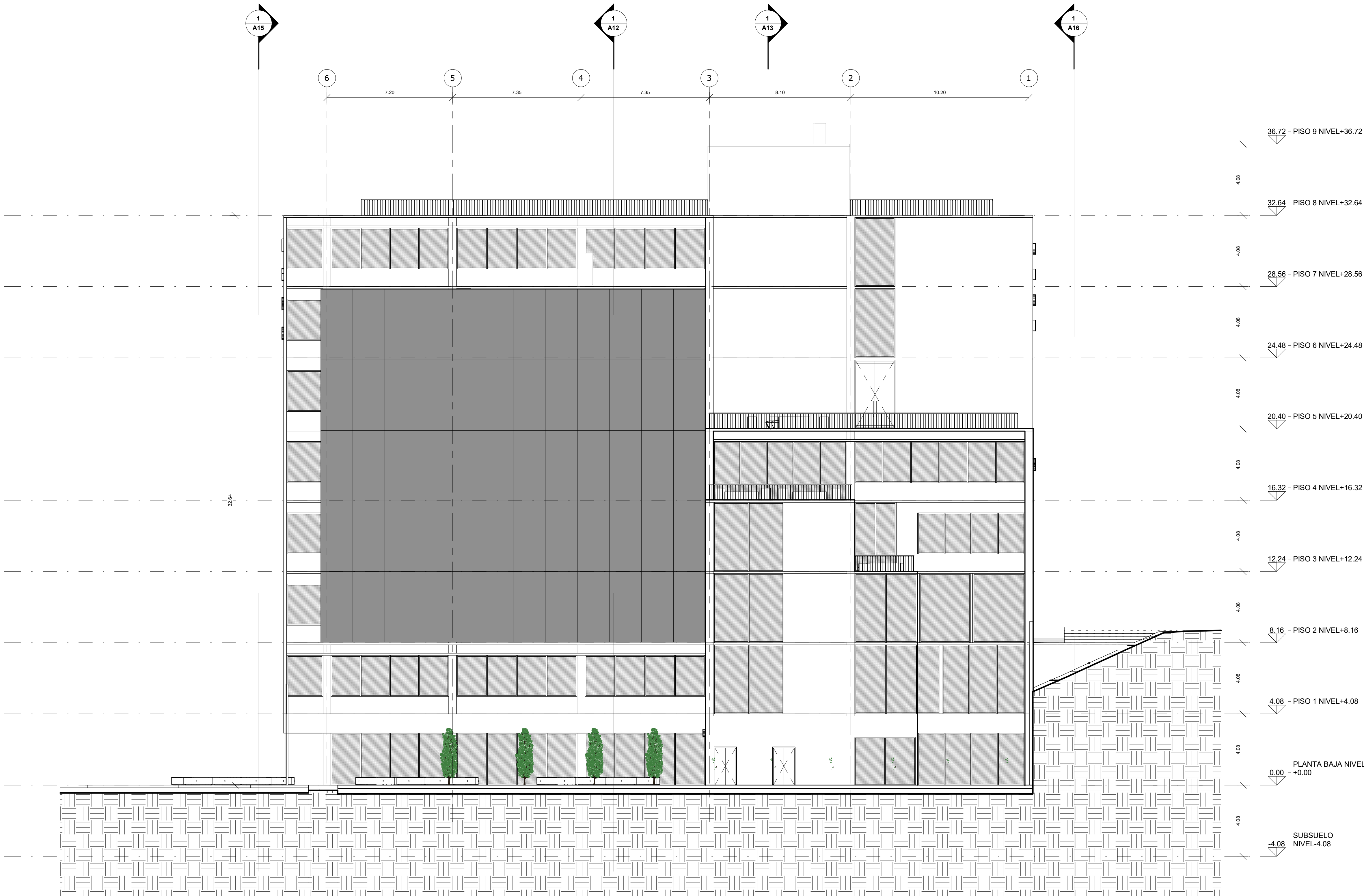
1 Sección 7 1 : 125
