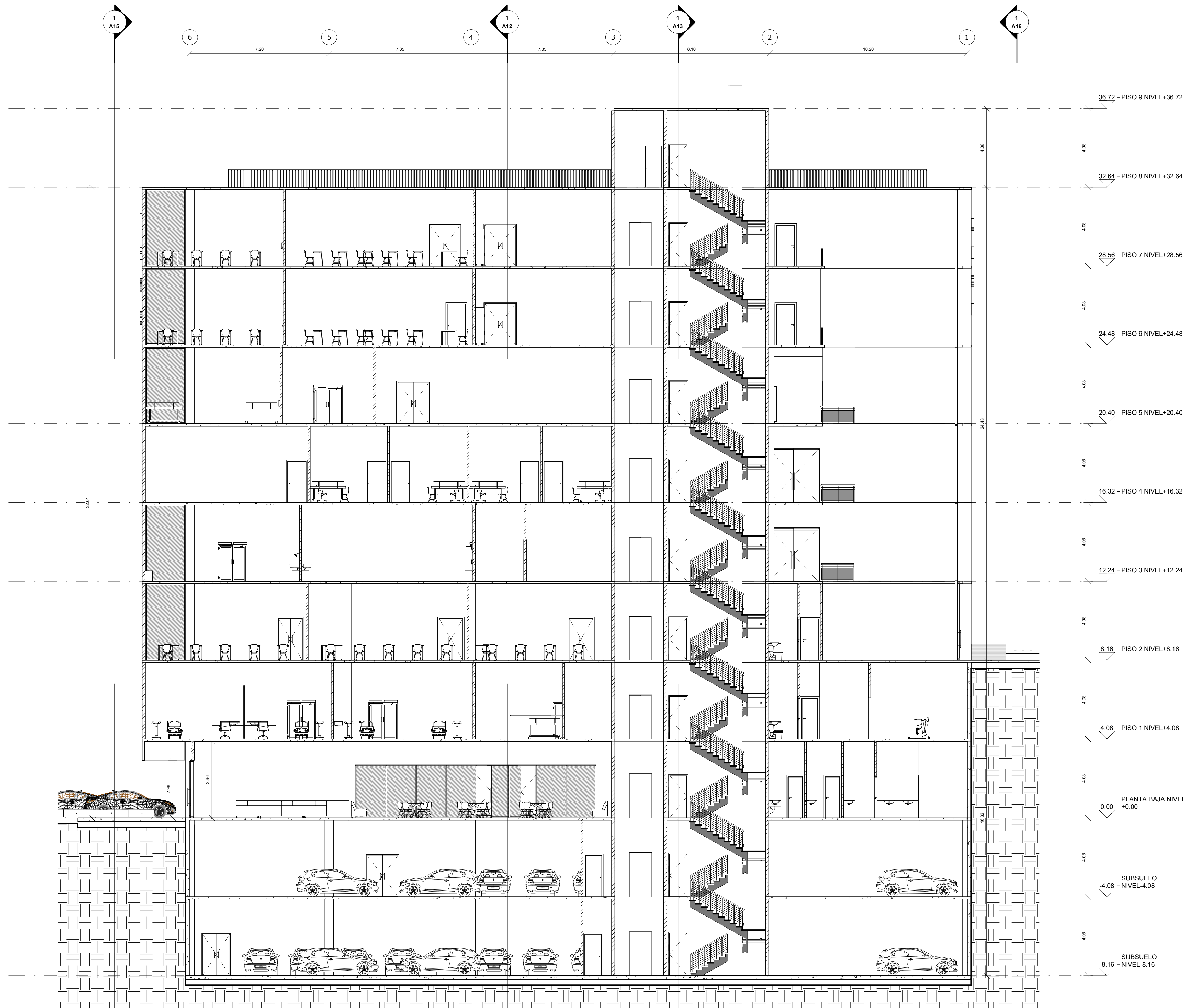
1 Sección 3 1 : 100
