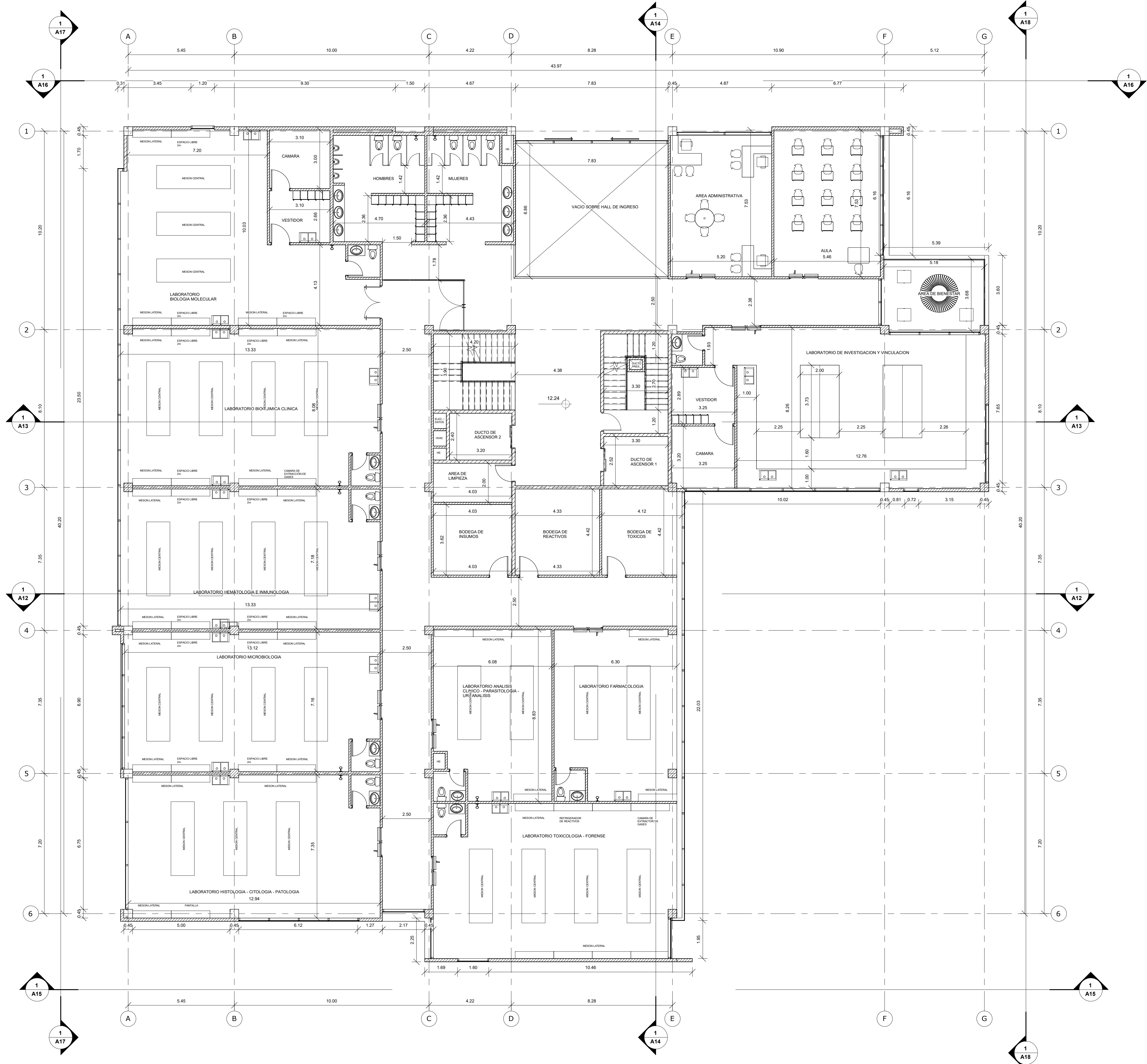
1 PISO 3 NIVEL+12.24 1 : 100
