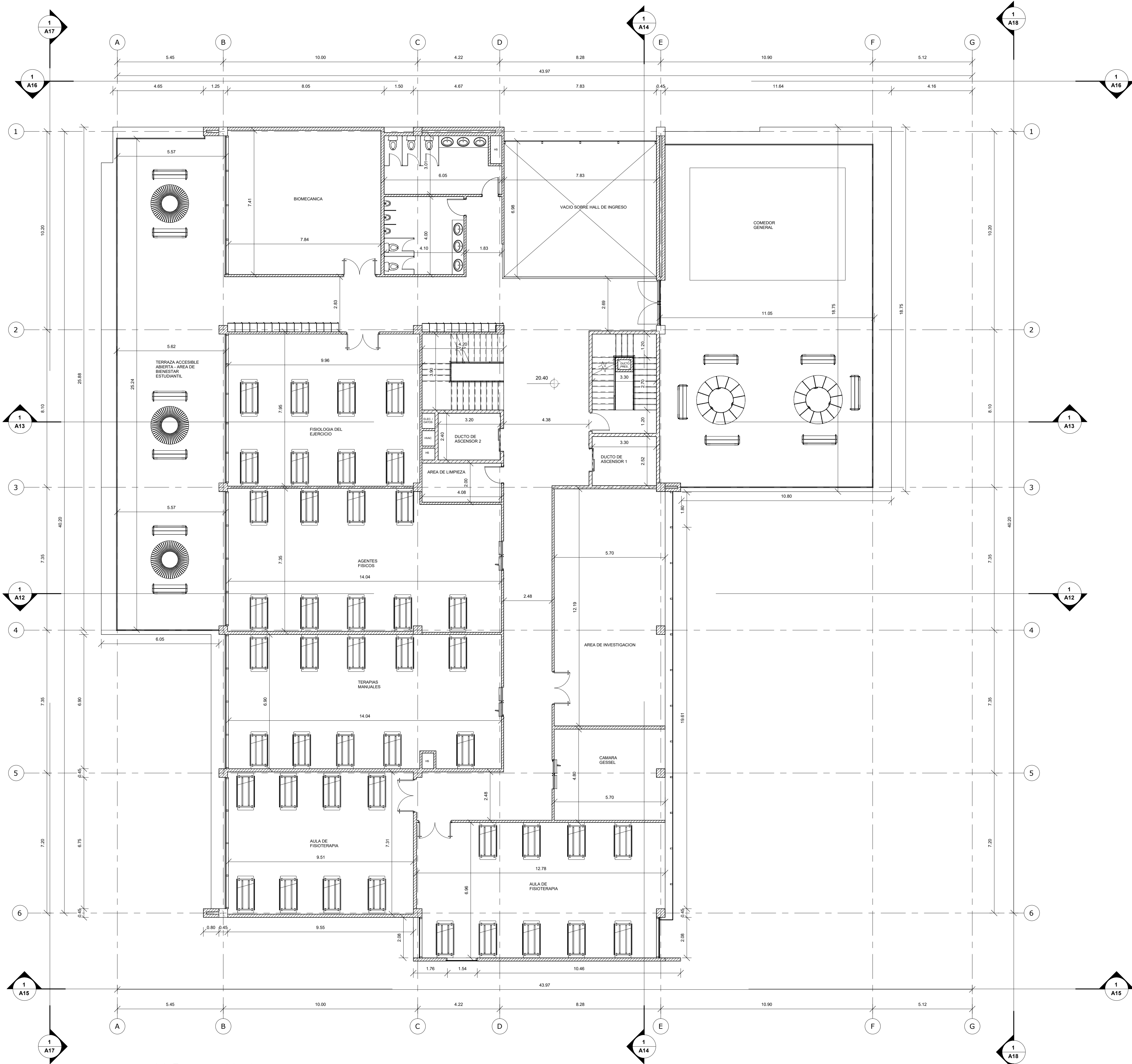
1 PISO 5 NIVEL+20.40 1 : 100
