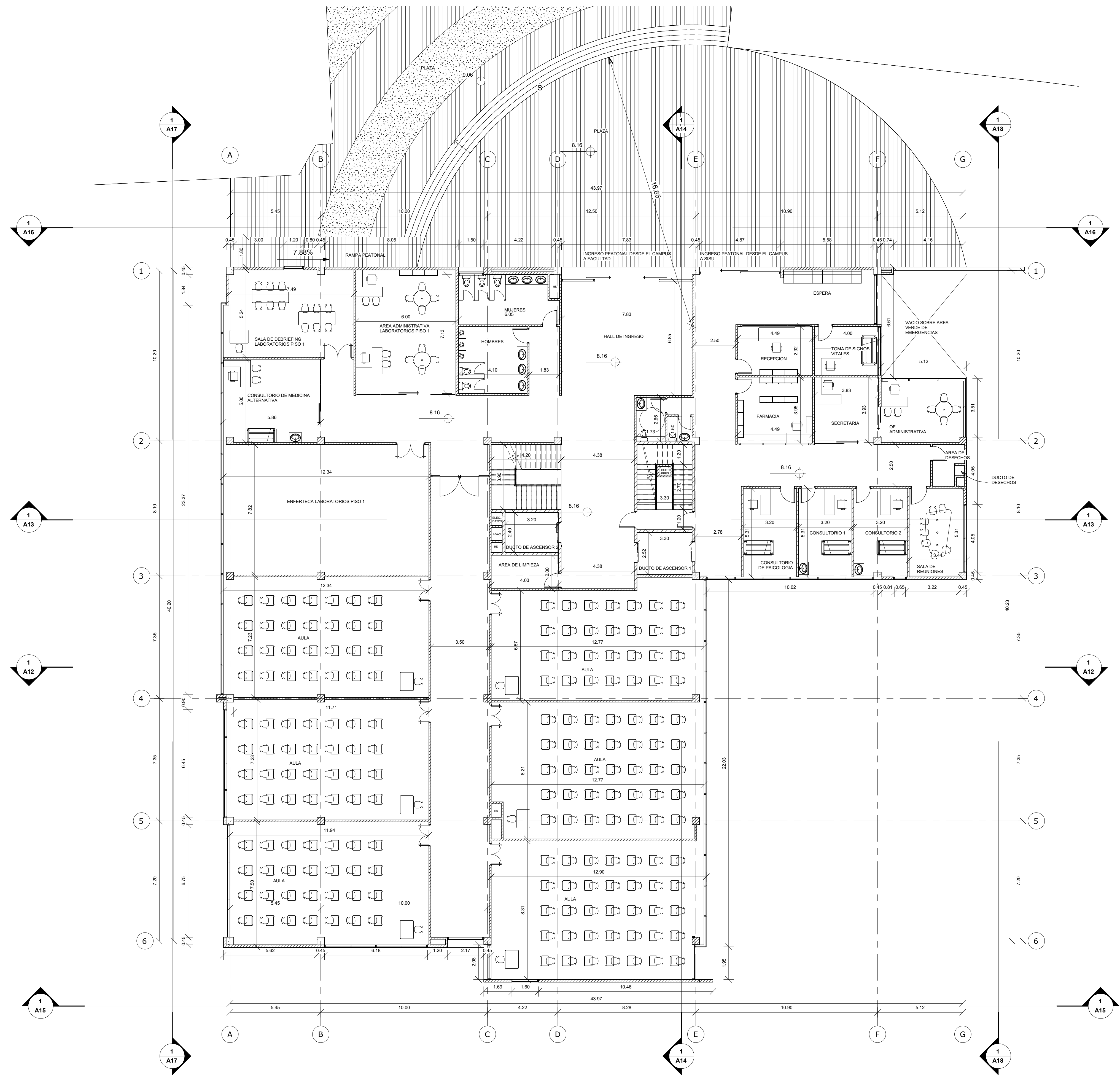
1 PISO 2 NIVEL+8.16 1 : 125
