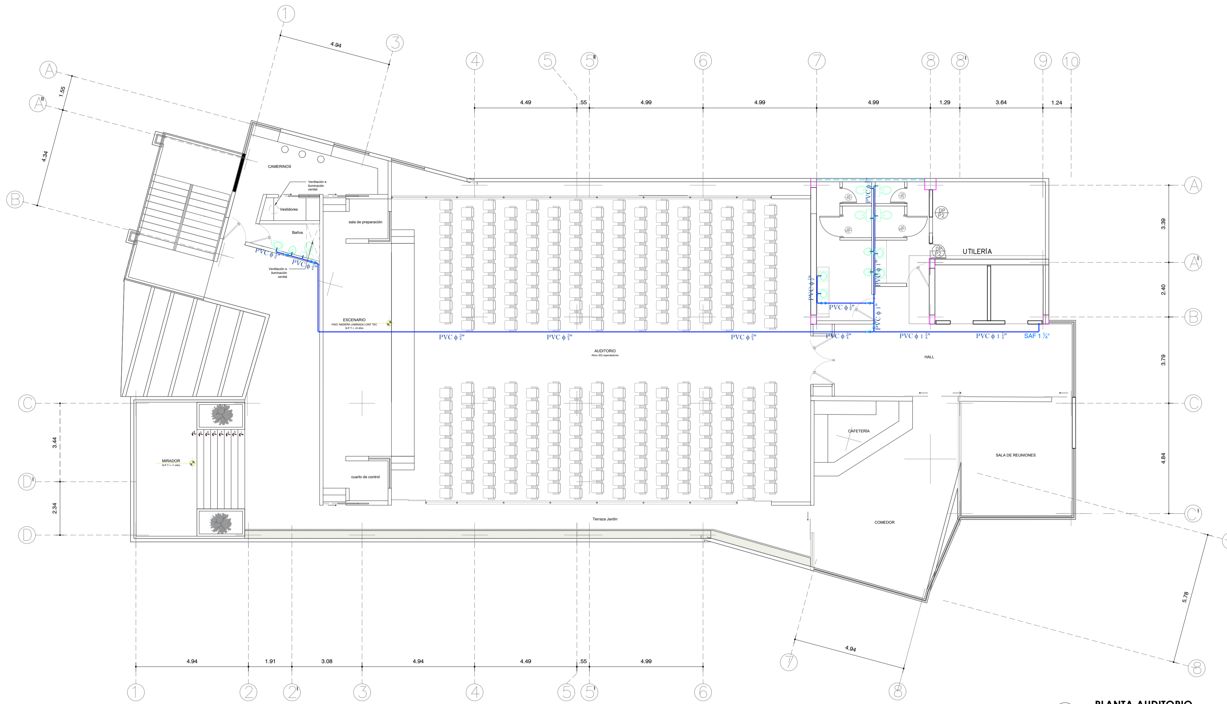
PLANTA AUDITORIO ESC: 1/100
