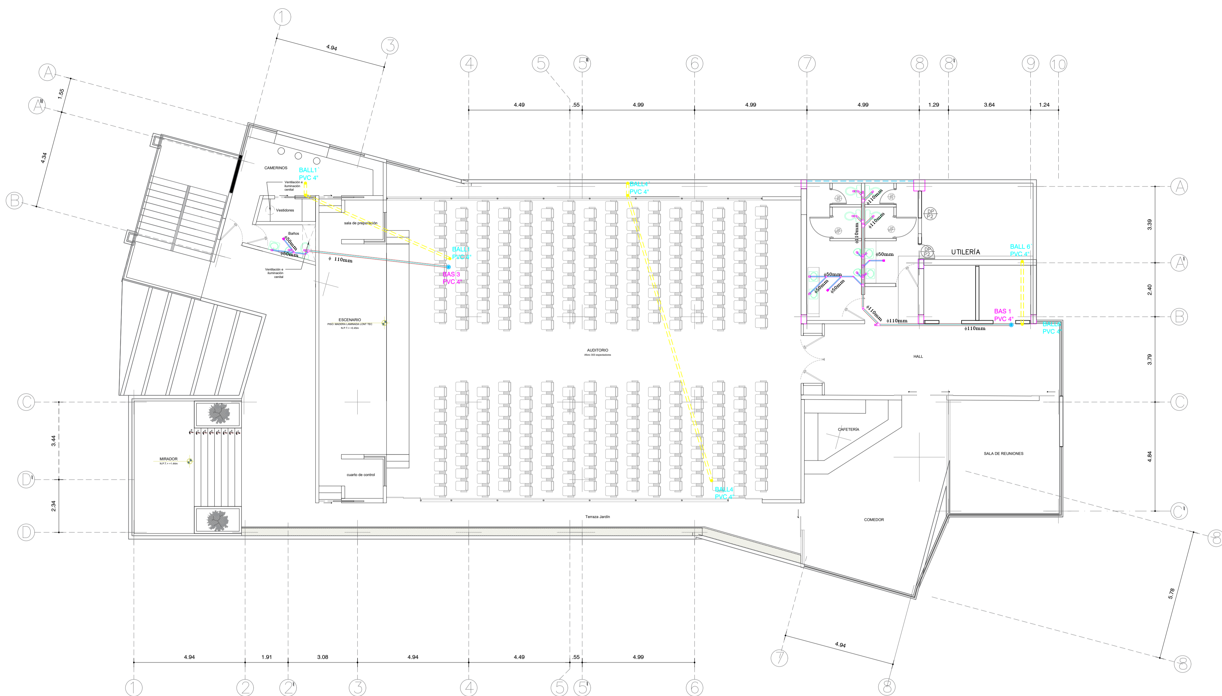
8 PLANTA AUDITORIO ESC: 1/100
