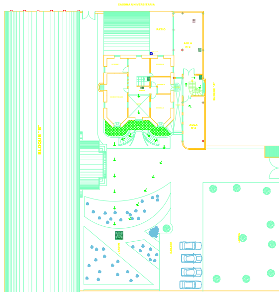
SEGUNDA PLANTA
