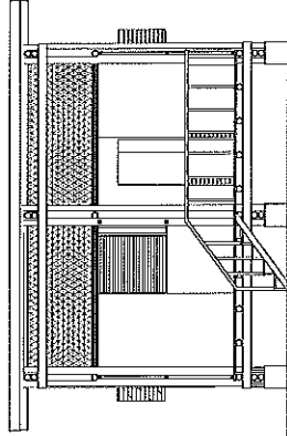
FACHADA OESTE ESCALA: 1:50
