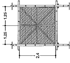
MODULACIÓN ESCALA: 1:50
