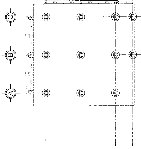
CIMIENTO ESCALA: 1:50
